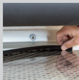
4 / Insérer le joint de vitrage supérieur.
