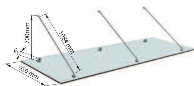
3 haubans pour longueurs : 2000-2400 mm
