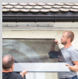
2 / Enficher le profilé de protection des arêtes sur le verre (respecter le sens) et insérer ensuite la vitre dans le profilé de la marquise en plaçant les trous de perçage en bas.
